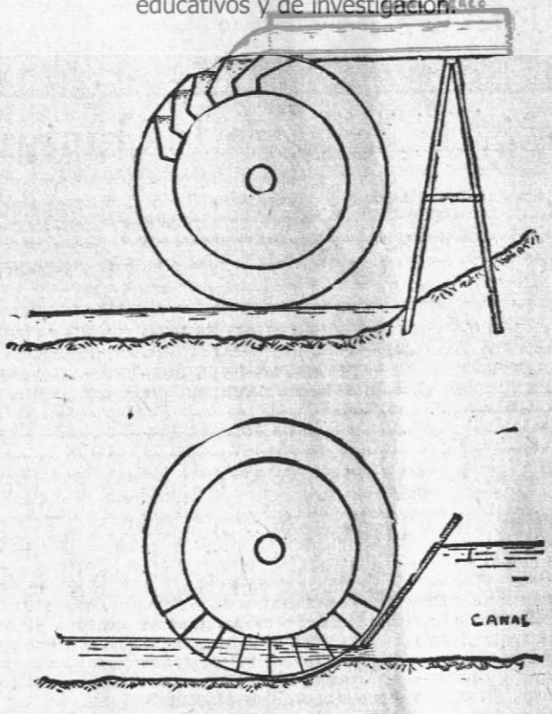
A. Esquema de rueda hidráulica con canal inferior. B. Esquema de rueda hidráulica con canal superior.
